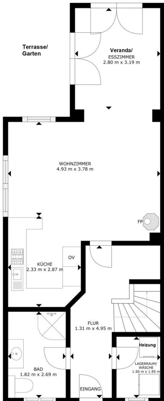
Grundriss-Erdgeschoss
